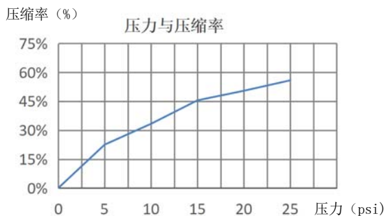
压缩曲线图 (2.0mm)
