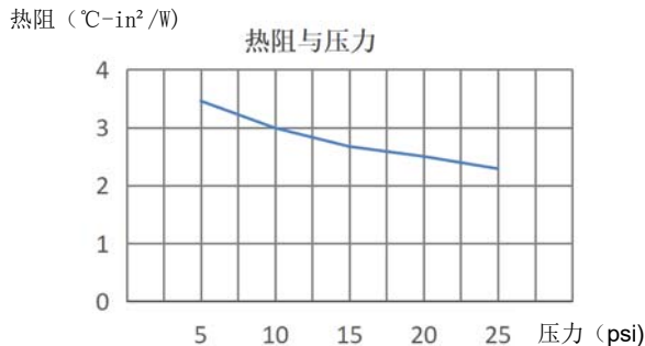
热阻曲线图
